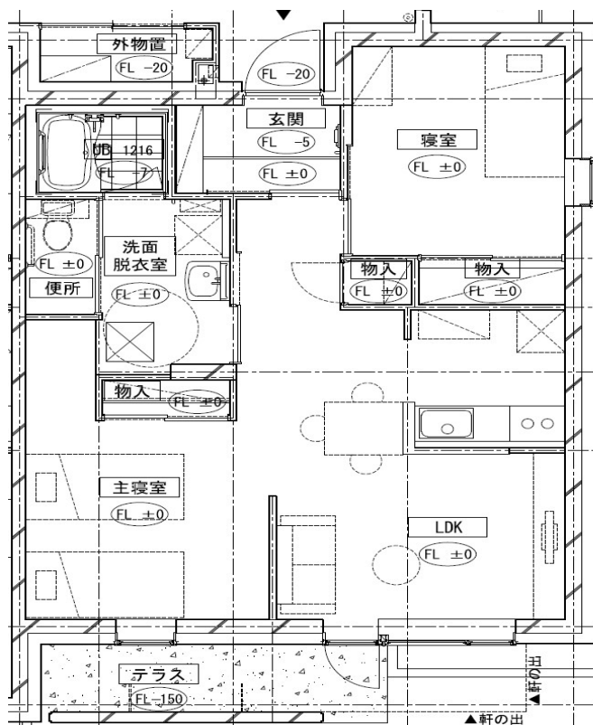
③間取り
