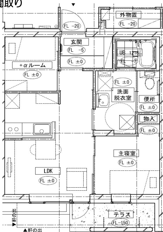
①間取り
