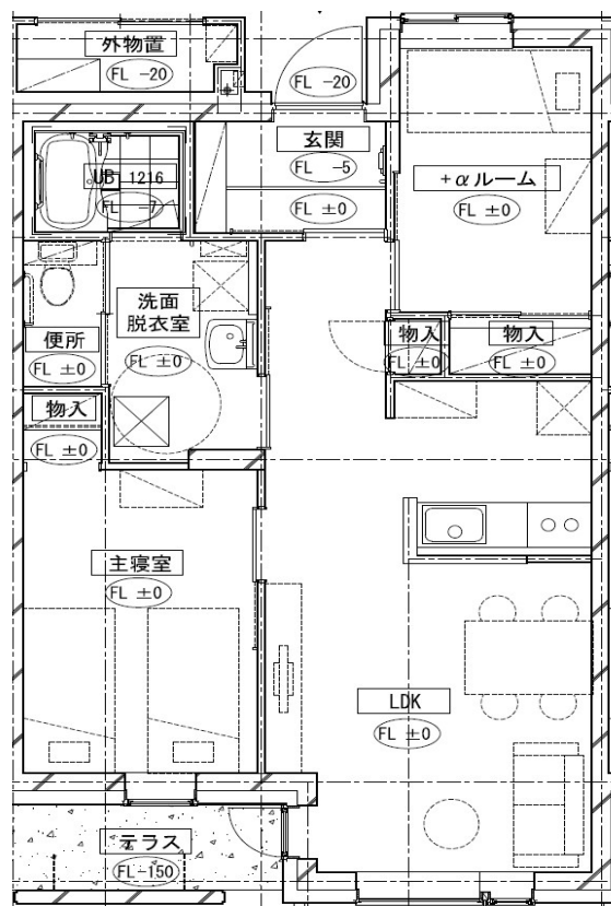
②間取り
